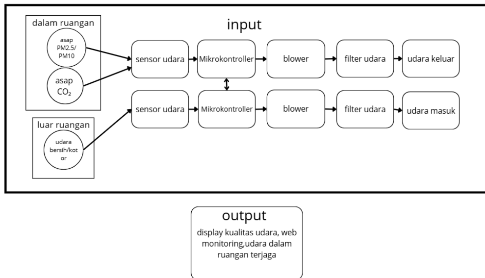
Gambar 1.1 Sistem Kerja Alat
