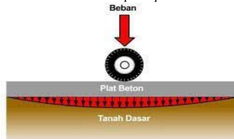
Gambar 1.2. Distribusi Beban pada perkerasan Lentur dan Kaku.
